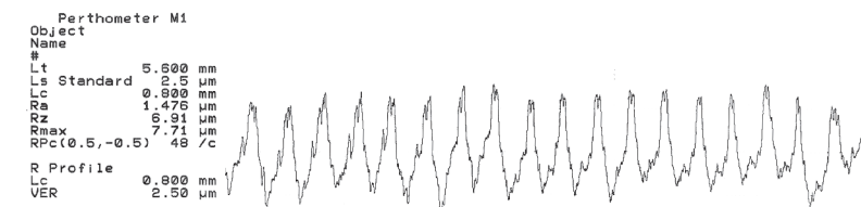
平面粗さ
